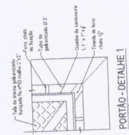
19 PORTÃO - DETALHE 1 1:75
